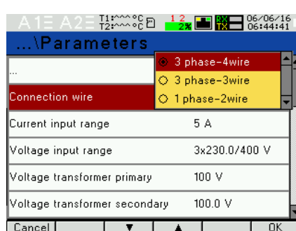
Fig. 15. Screens of Parameters mode
