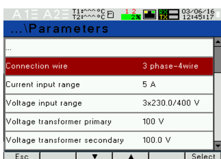
Fig. 15. Screens of Parameters mode
