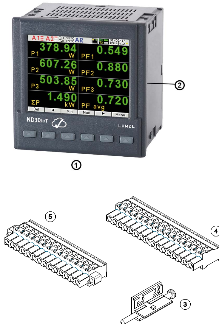
Fig. 1. Meter set
